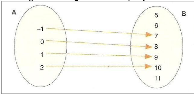
Figura 2: Diagrama da relação y = x + 8
