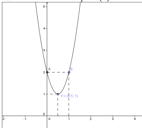
Figura 14: Gráfico da função h(x) = 4x^2 - 4x + 2
