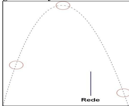
Figura 8: Trajetória da bola de vôlei
