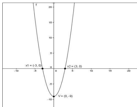
Figura 12: Gráfico da função f(x) = x^2 - 9
