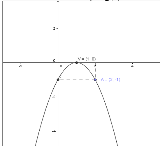
Figura 13: Gráfico da função g(x) = -x^2 + 2x - 1
