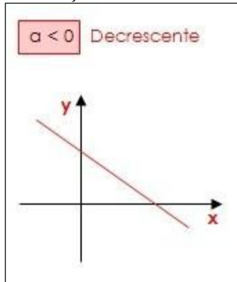
Figura 6: Função Afim – Decrescimento
